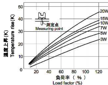
温度上昇(参考)MQS,MQR Temperature rise(ref.)MQS,MQR
