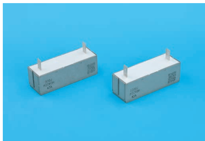
预充电阻 (超高耐用性和高压兼容性)
