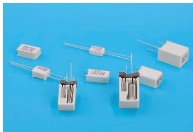
小型高耐冲击防止电阻器 (配有热熔断器和热敏电阻)
