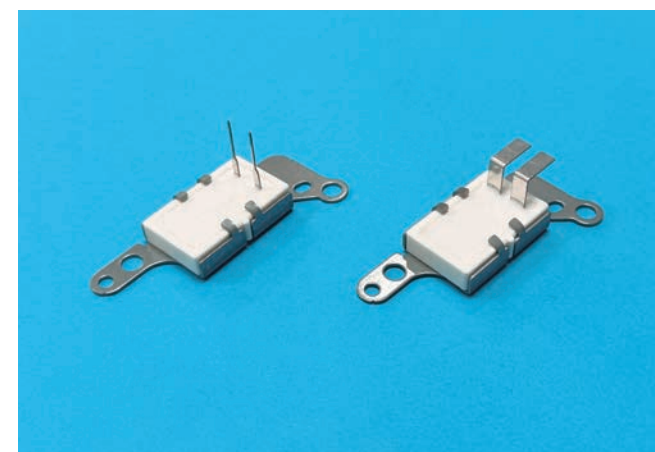
泄放电阻 (直接附着型)
